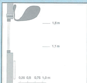
Spridningsbild från sidan Luftflöde: 8l/s Rumstemperatur: +20° Tilluftstemperatur: -20° Radiatoreffekt: 750W
