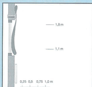
Spridningsbild från sidan Luftflöde: 8l/s Rumstemperatur: +20° Tilluftstemperatur: +/-0° Radiatoreffekt: 400W
