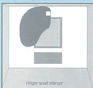
Spridningsbild framifrån Luftflöde: 6l/s Rumstemperatur: +20° Tilluftstemperatur: +/-0° Radiatoreffekt: 400W
