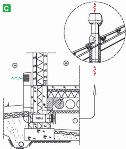
第4種換気の給気
