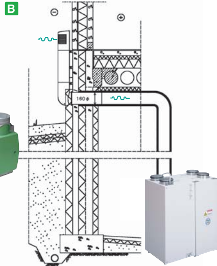
熱交換の給気
