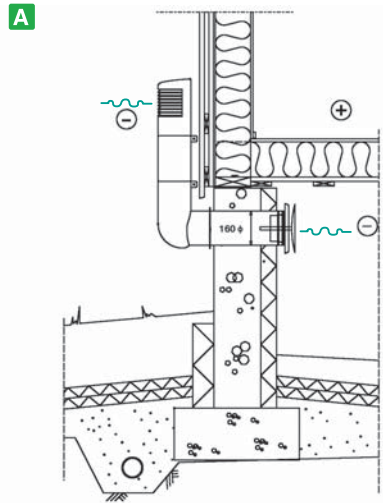
排気!! 給気!!
